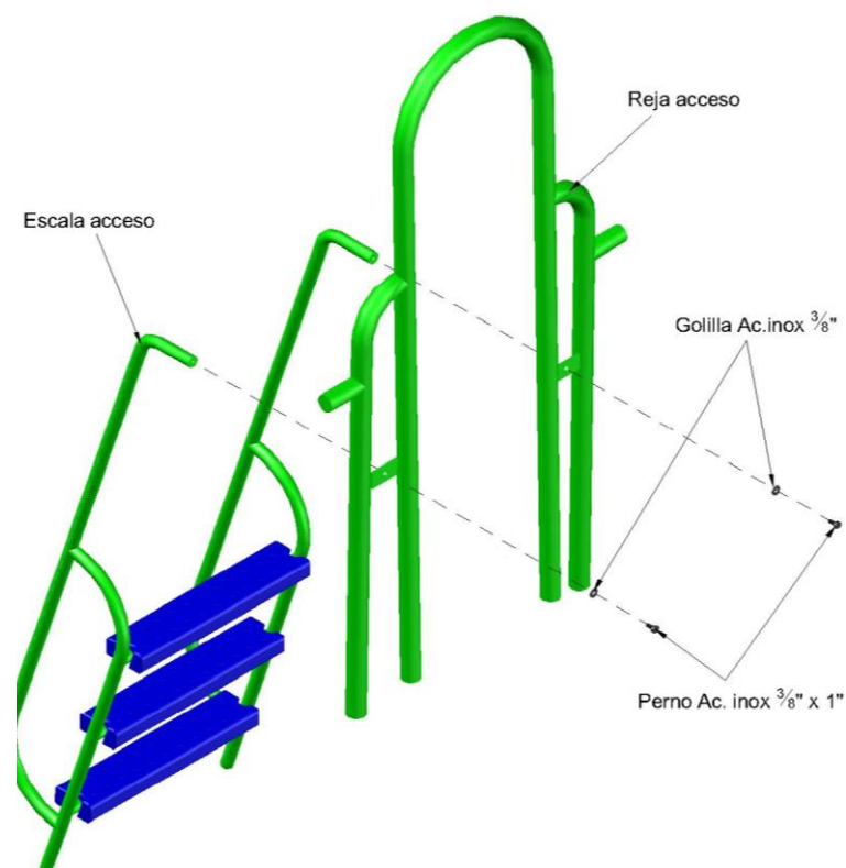
Escala Acceso a Reja Protección
