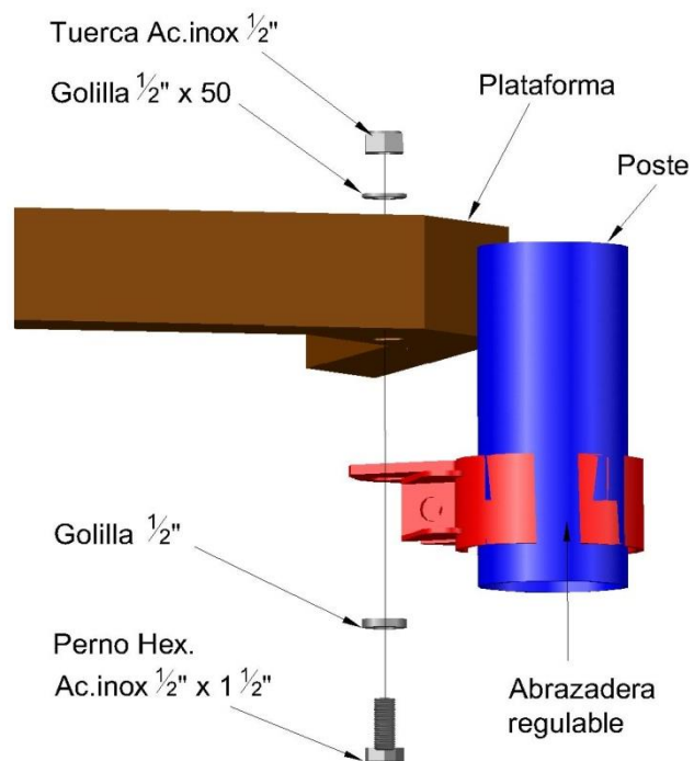
Soporte de Plataforma a Poste
