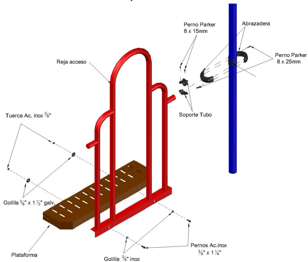
Escala a Reja de Acceso
