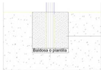
Fundación de hormigón. H25 Clase 4
