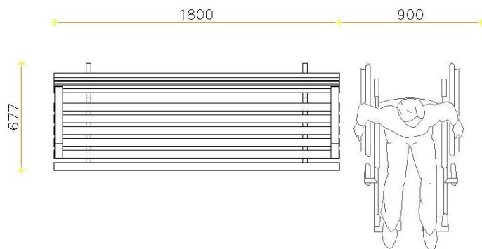
PLANTA
