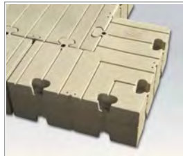
Utility channel, outside corner 8024371 Beige ⊕ 0,5 x 0,5 x 0,4
